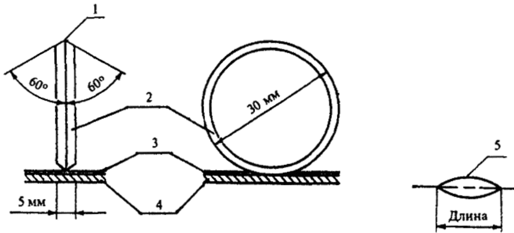
1 - острый край; 2 - индентор; 3 - покрытие; 4 - основание; 5 - форма отпечатка
