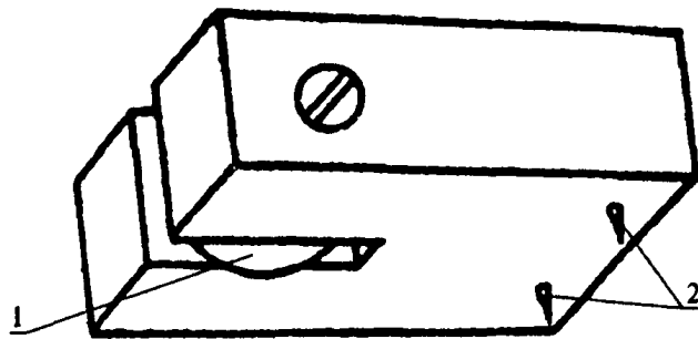
1 - индентор; 2 - опоры
