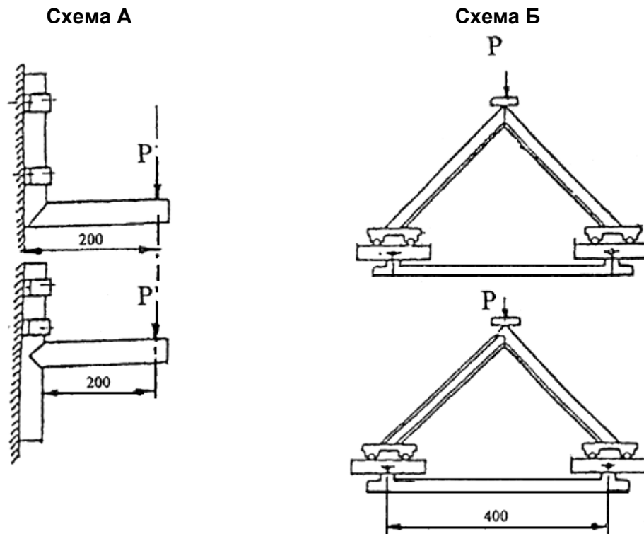
Рисунок 4 - Определение прочности угловых сварных соединений (для углового соединения под 90° и Т-образного соединения)
