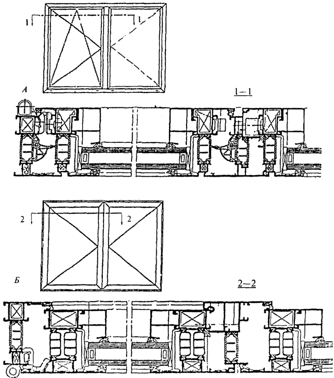
Рисунок 6 - Примеры конструктивных решений срединного притвора
